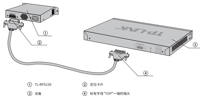
图3-5 连接设备和TL-RPS150示意图
