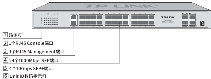
图1-2 TL-SH6428F前面板示意图
