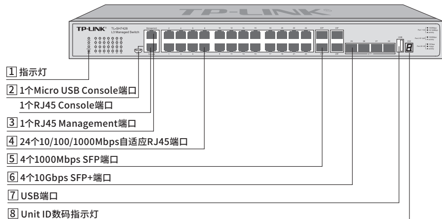
图1-3 TL-SH7428前面板示意图
