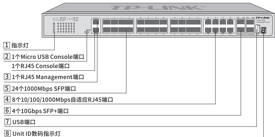
图1-4 TL-SH7428F前面板示意图
