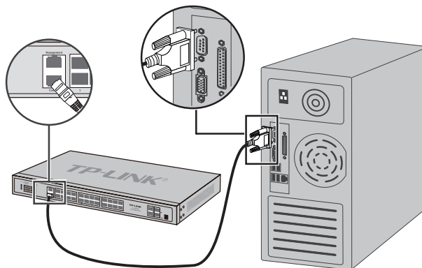
图3-2 RJ45 Console端口连接示意图
