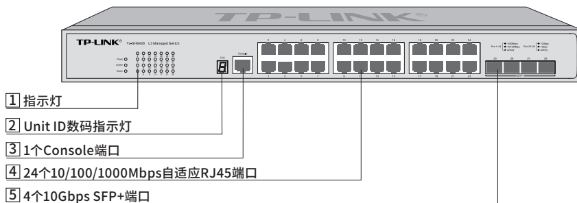
图1-1 TL-SH6428前面板示意图
