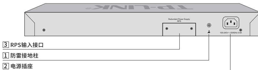
图1-7 TL-SH7428/TL-SH7428F后面板示意图
