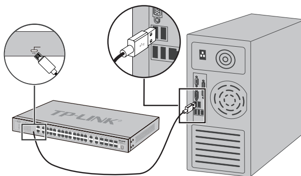
图3-3 Micro USB Console端口连接示意图
