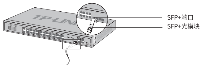
图3-1 SFP+端口连接示意图
